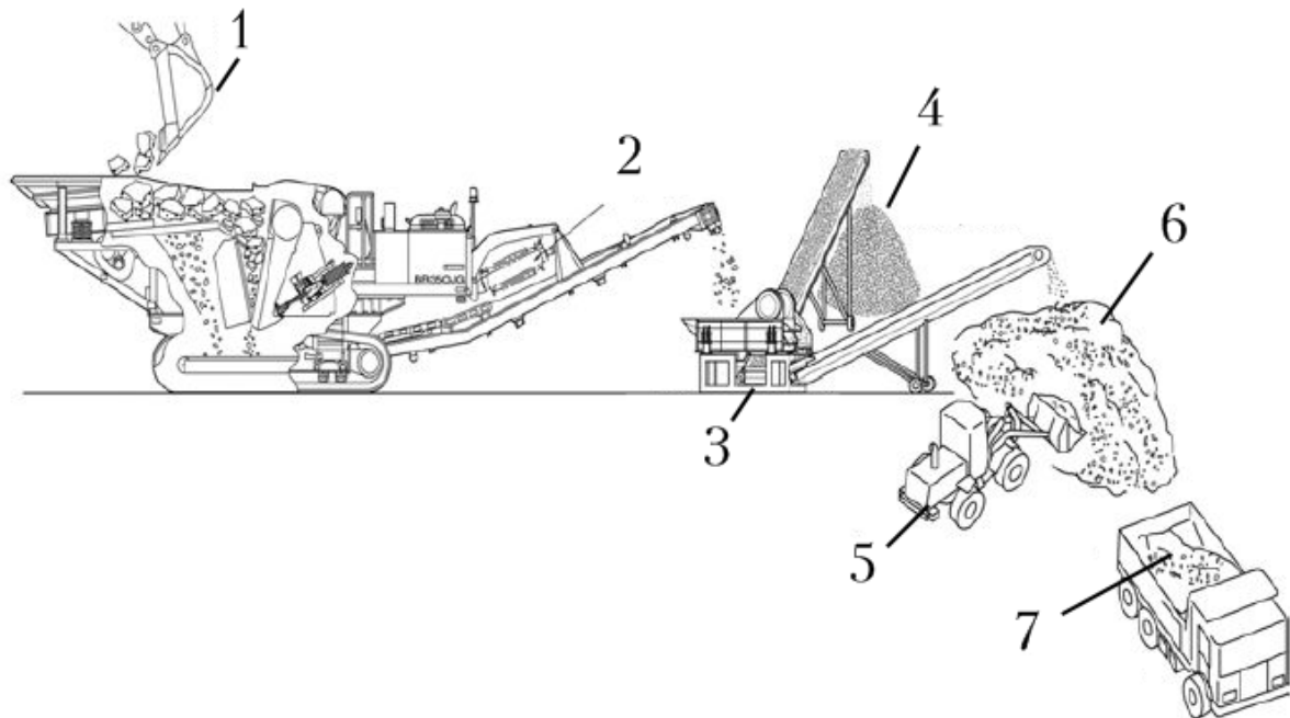
Рисунок 5.1 – Схема подрібнення будівельних відходів
