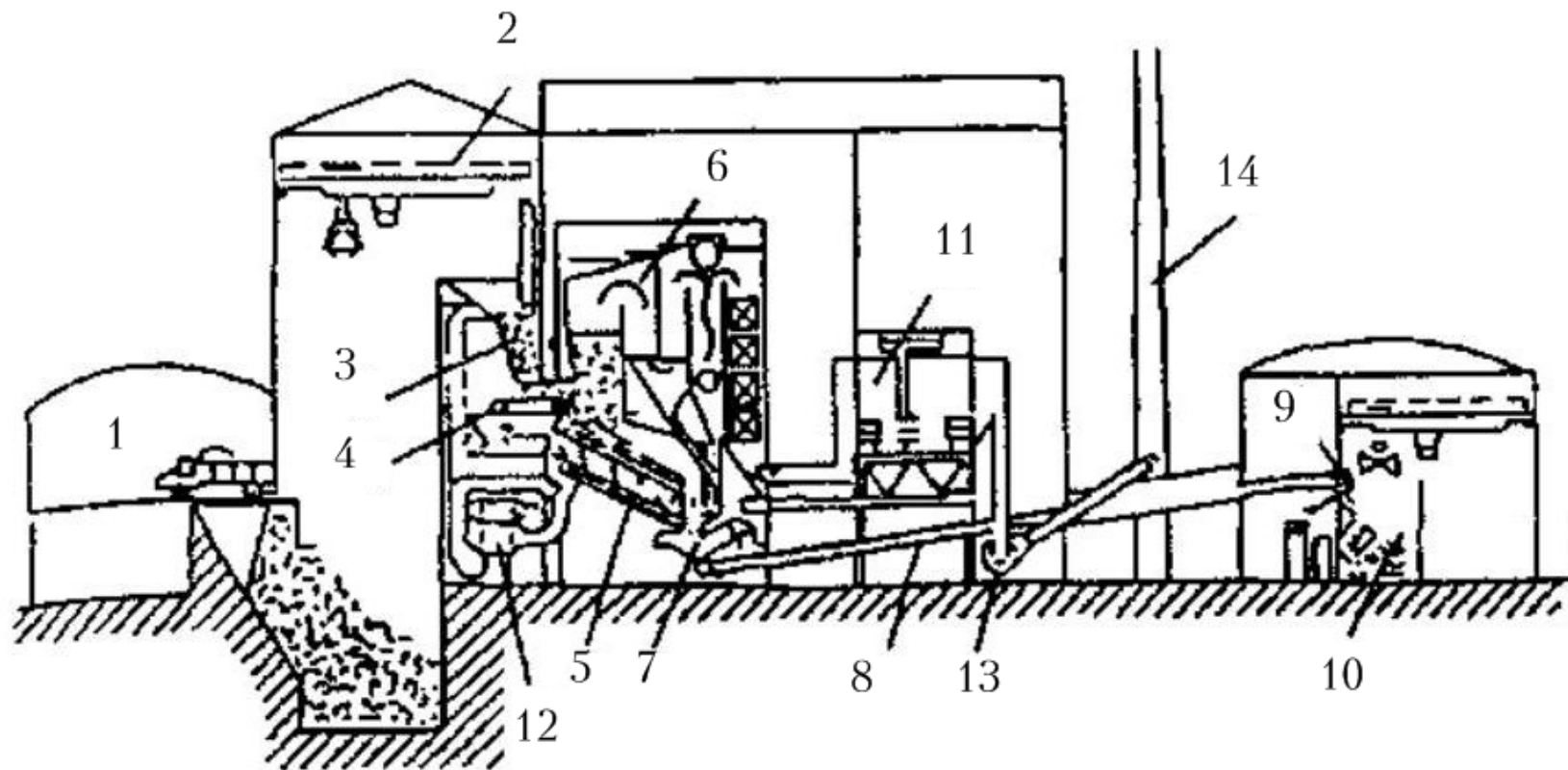
Рисунок 9.13 – Технологічна схема сміттєспалювального заводу
