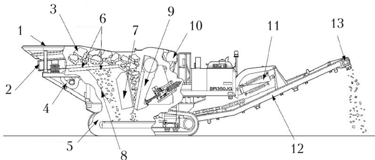
Рисунок 5.2 – Подрібнювач будівельних відходів
