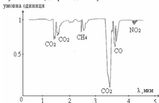
Рис. 1. Коливально-обертальні смуги поглинання димового газу ІЧ випромінюванням
