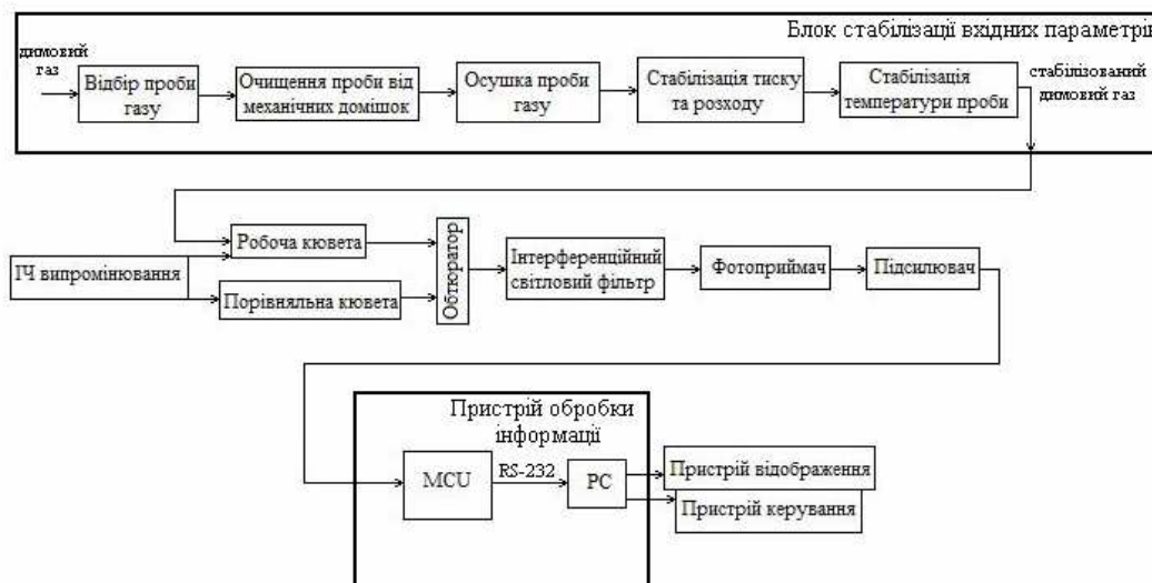
Рис. 4. Функціональна схема системи контролю складу димового газу котельних установок
