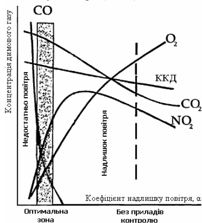
Рис. 3. Структура складу димових газів котельних установок
